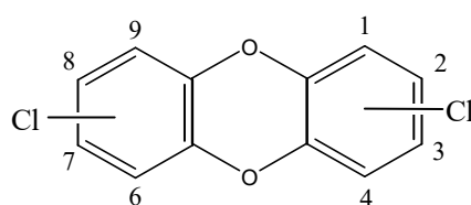
PCDDs の構造
